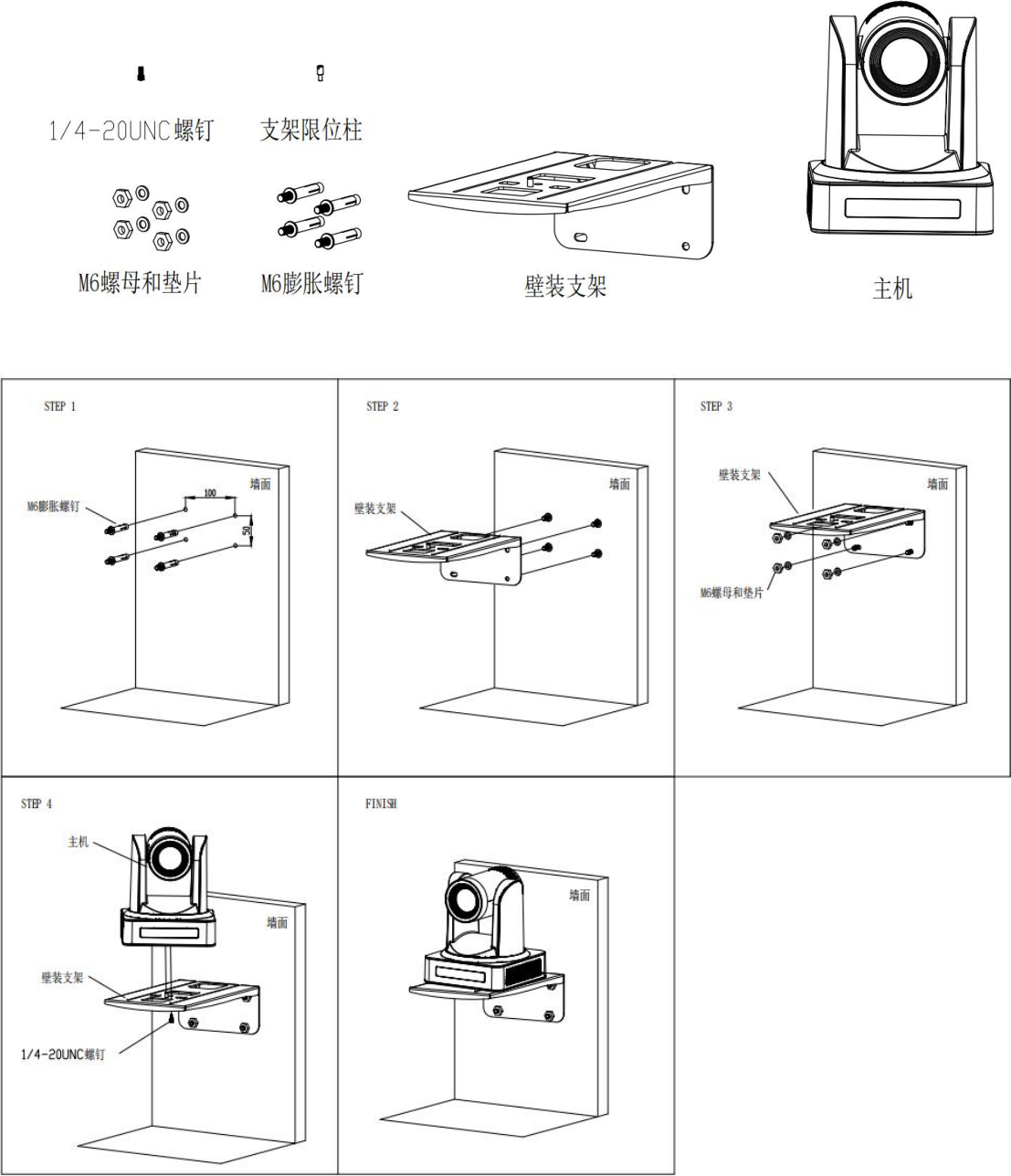
图 1-2 支架正装步骤
