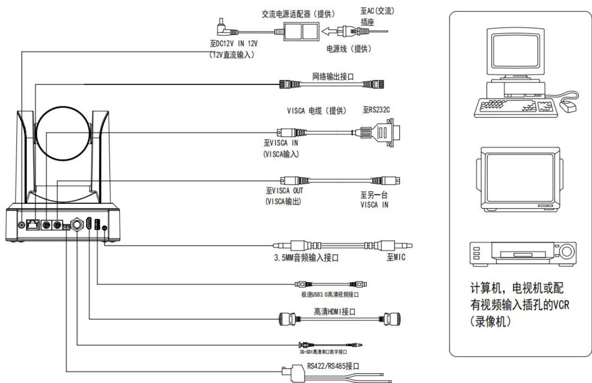
图 2-2 外部接口示意图
