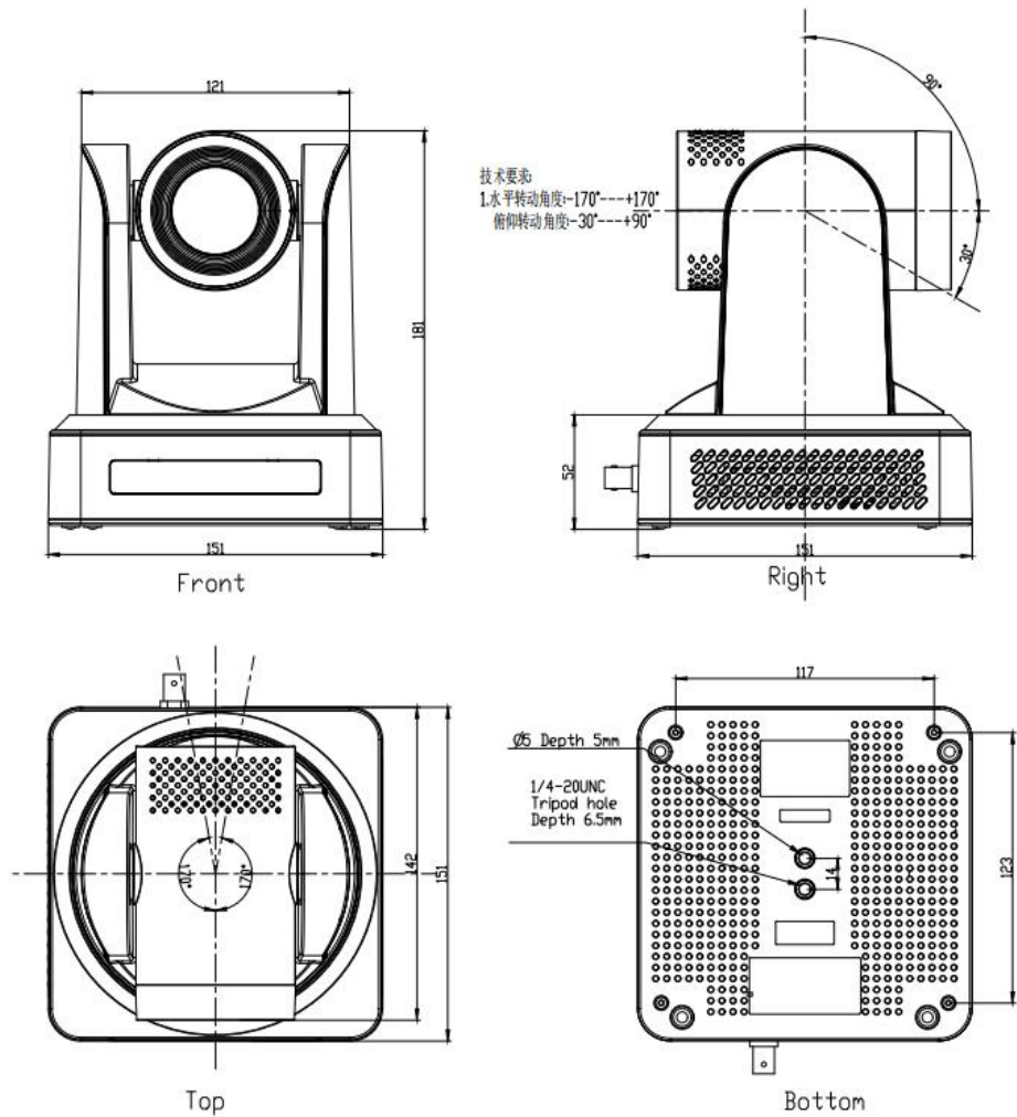
图 2-1 外型尺寸
