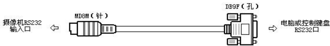
图 2-3 RS-232 接口示意图
