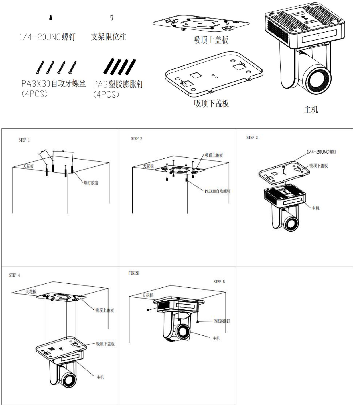
图 1-3 支架倒装步骤
